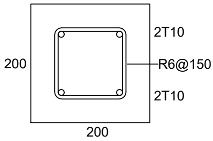
STIFFENER COLUMNS
