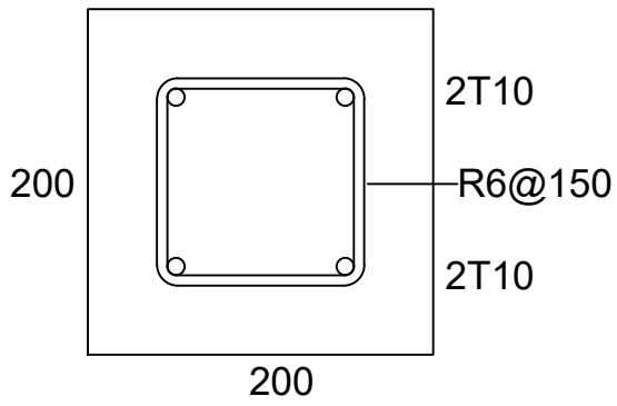
STIFFENER COLUMNS
