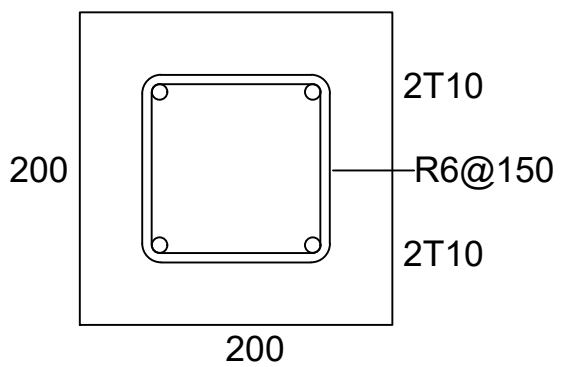
STIFFENER COLUMNS
