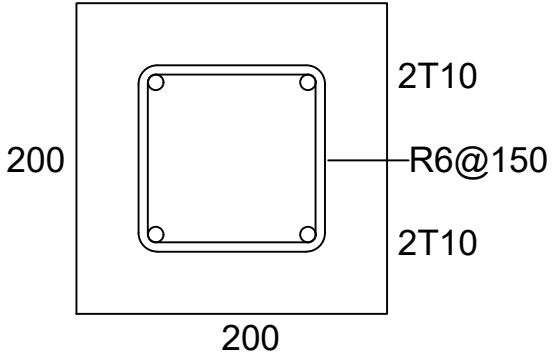
STIFFENER COLUMNS
